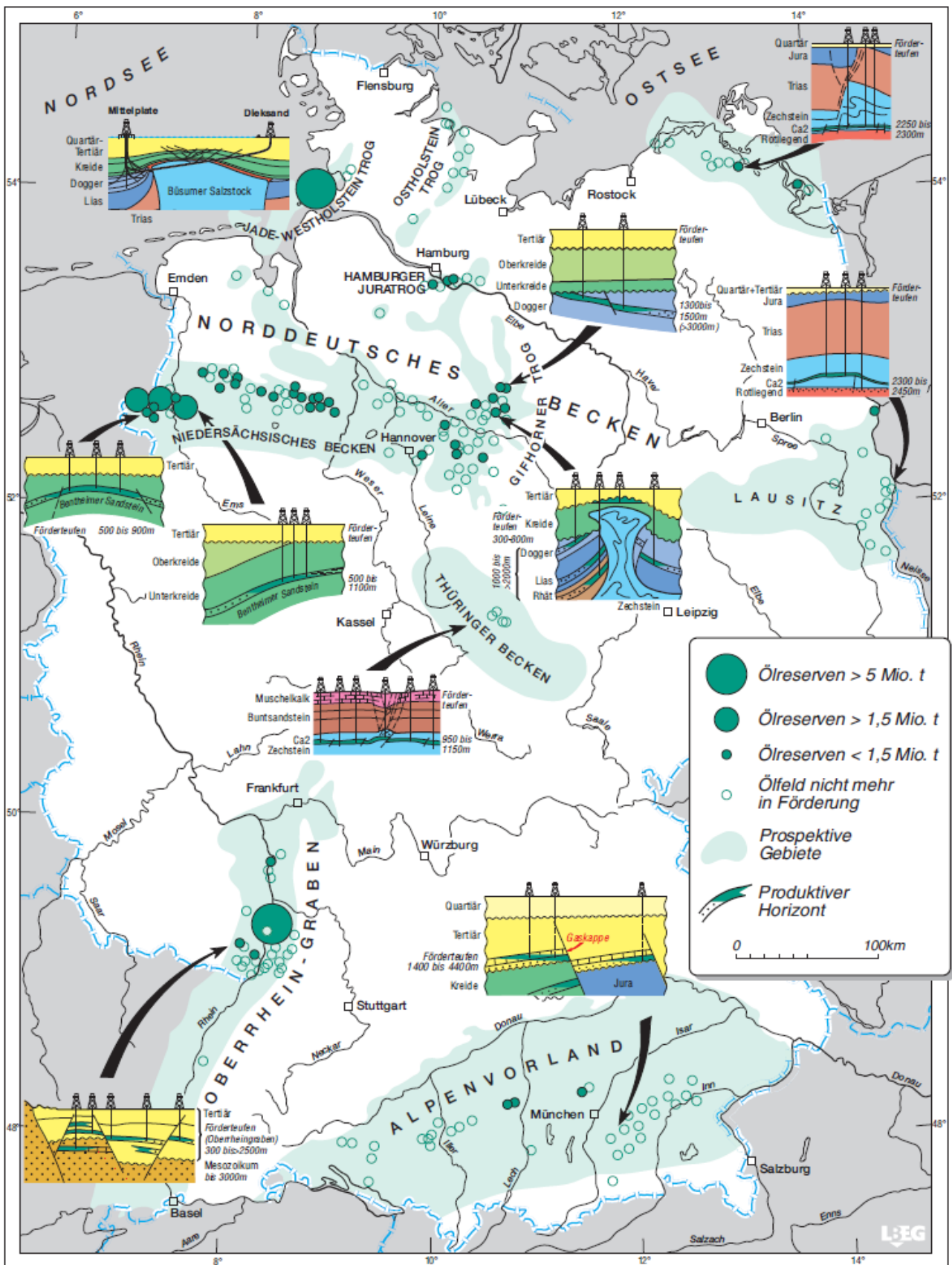
Prospektive Gebiete, Erdölfelder und charakteristische Erdölstrukturen.
