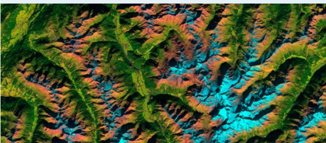
Aufnahme der Ötztaler Alpen (Tirol, Österreich) vom Copernicus Sentinel-2a-Satelliten am 16. Oktober 2016
