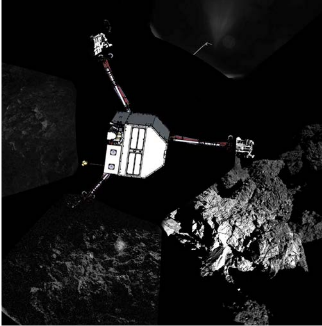
Das CIVA-Kamerasystem stellte das erste Panoramabild der Kometenoberfläche mit Philaes Position zur Verfügung. Es zeigt eine 360-Grad-Ansicht der Landestelle.
