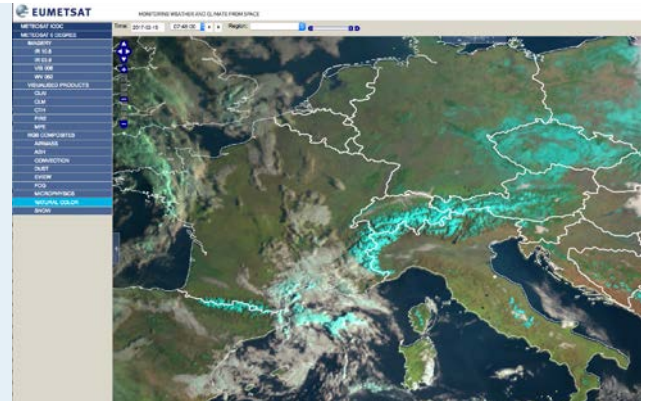
EUMETSAT-Aufnahme mit „Natural Color“
